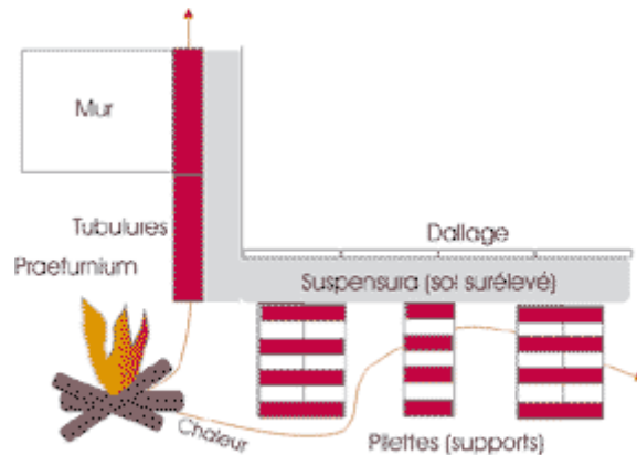
Coupe d'un hypocauste. Dessin d'après JP Adam 1994
